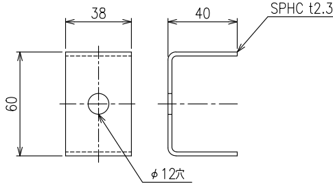
コの字部詳細
